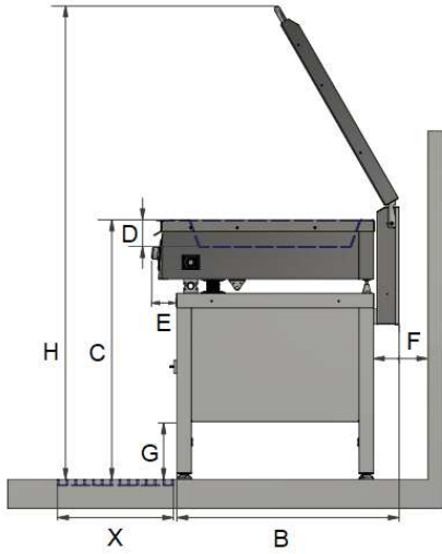
Alle mål i mm
